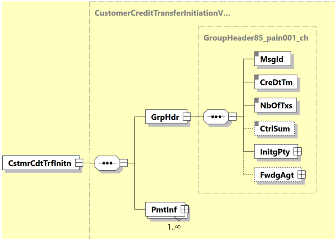
Abbildung 11: Group Header (GrpHdr)
