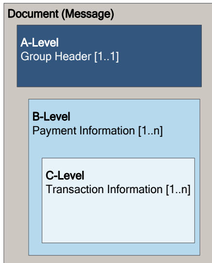
Abbildung 4: Grundsätzliche Nachrichtenstruktur der XML-Meldung «pain.001»
